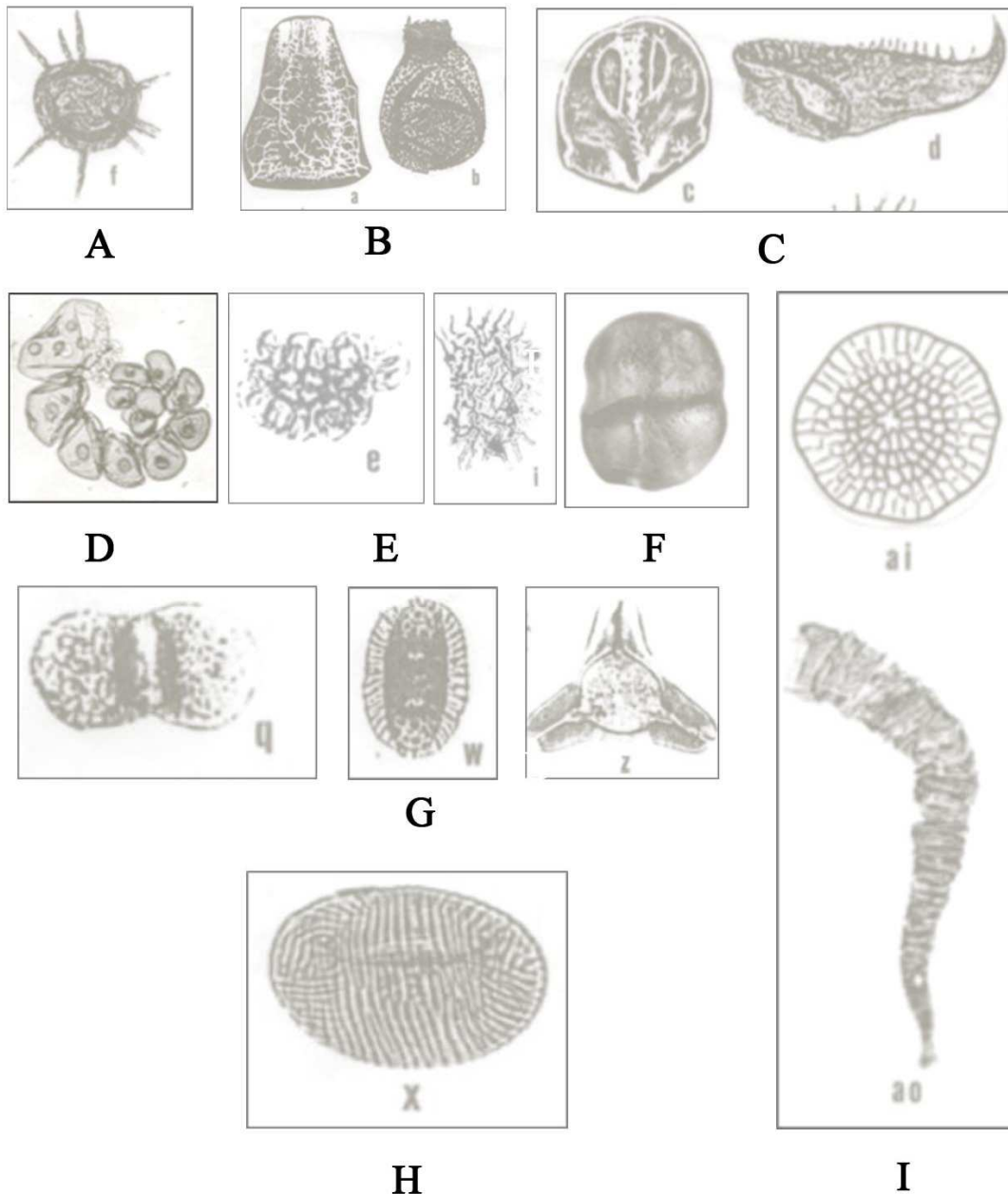
Figura 1. Palinomorfos. A. Acritarcas, Baltisphaeridium sp. R.W. Hedlund. B. Chitinozoa. a. Herochitina sp. W.A.M. Jenkins. b. Kalochitina multispinata R.W. Hedlund. C. Escolecodontos c. Xanthoprion albertensis J. Jansonius. d. Arabellites sp. R.W. Hedlund. D. Microforaminíferos. E. Microalgas, colonias de algas. e. Botryococcus sp. i. Pediastrum sp. F. Cryptoespora, cf. Pseudodyadospora sp. G. Polen. q. Pityopollenites pallidus Reissinger Nilsson. w. Wodehouseia spinata Stanley. z. Nudopollis sp. C.J. Félix. H. Esporas embriofíticas. x. Schizaeoisporites sp. R.W. Hedlund. I. Fungoesporas. Tomado de Traverse (1988).
