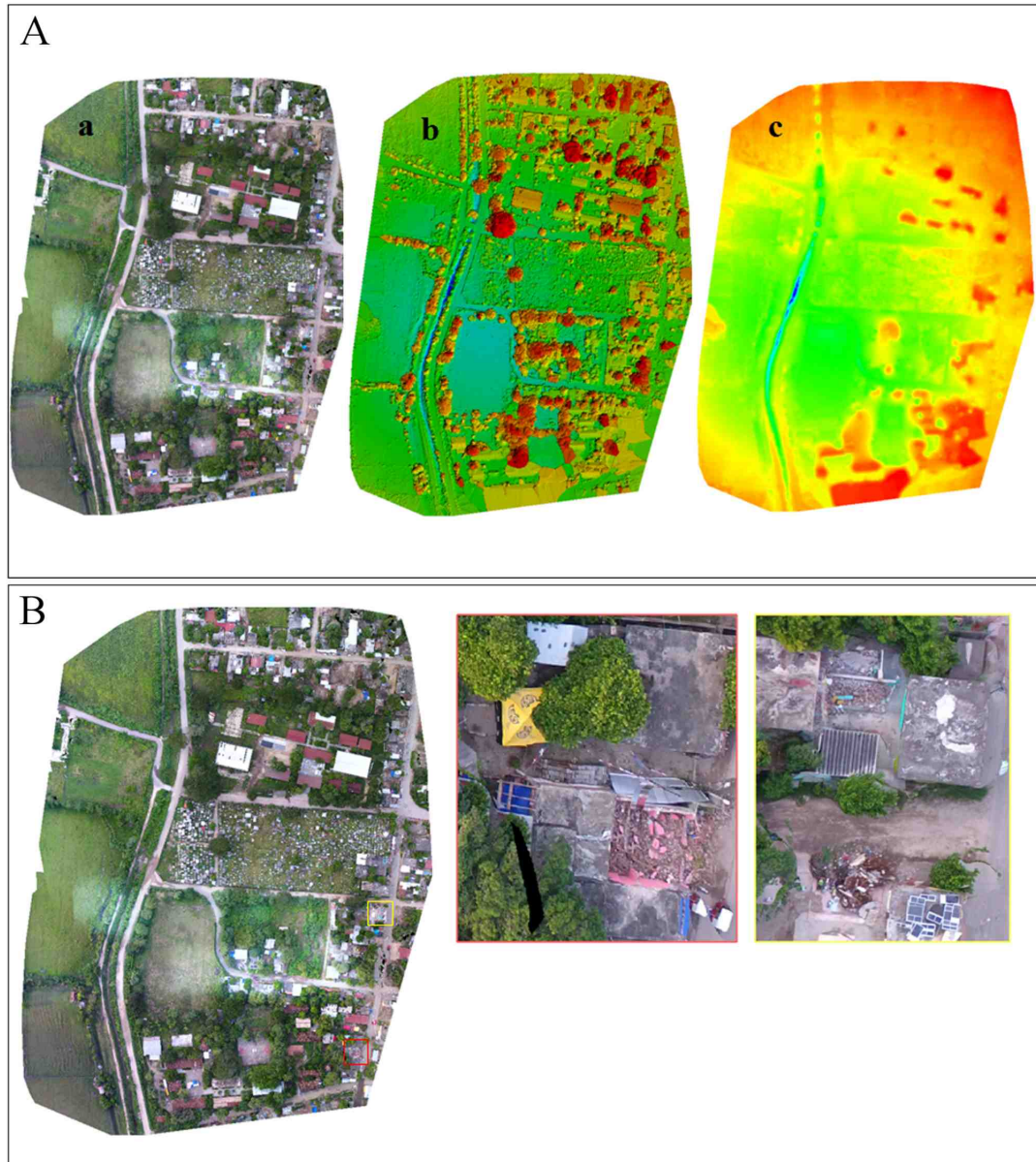
Figura 4. A. Zona del vuelo #1 correspondiente a la escuela Marista, ubicada en Asunción de Ixtaltepec, Oaxaca. a. Ortomosaico. b. Digital Surface Model (DSM). c. Digital Terrain Model (DTM). B. Mosaico y acercamiento a dos zonas con daño estructural, o derrumbes.
