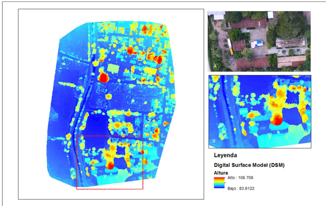
Figura 5. Digital Surface Model. A. Acercamiento a la zona de la escuela. B. Acercamiento a la misma zona en el DSM. Es importante señalar que las unidades de las alturas pueden variar sin embargo, suelen ser representadas por unidades de metros sobre el nivel del mar (msnm).
