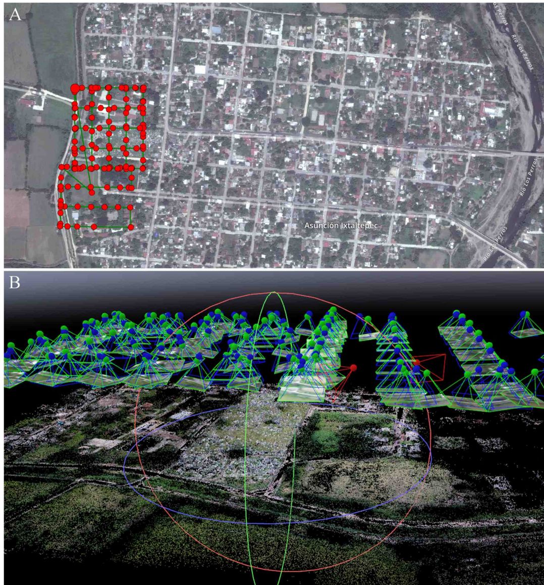
Figura 3. A. Ubicación del vuelo en Asunción Ixtaltepec y ruta de vuelo del dron. La ruta está trazada como un doble grid o doble gradilla, que utiliza las mismas líneas de vuelo en direcciones perpendiculares para asegurar el cruce por los mismos vértices. Esta técnica es útil para obtener varias imágenes del mismo punto (puntos rojos) y en diferentes ángulos. B. Vista lateral de la nube de puntos. Las pirámides verdes, azules y rojas representan las “cámaras” o las imágenes que fueron tomadas para cada punto. Las cámaras rojas, indican imágenes no procesadas debido a movimientos propios del dron, obstrucciones o fenómenos naturales (ráfagas de viento) que ocasionan movimiento inesperado y por tanto, imágenes movidas o borrosas, las cuales pueden prenderse o apagarse según sea conveniente.
